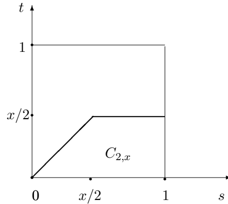
Рис. 4: Область C_{2x} , 0 < x \leq 2 .
