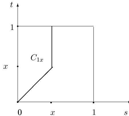
Рис. 3: Область C_{1x} , 0 < x \leq 1 .
